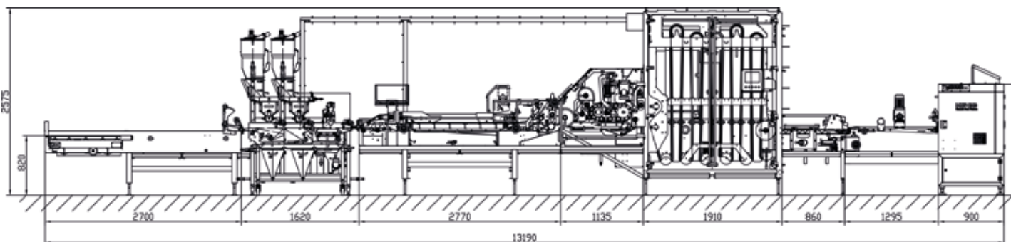
станция отсадки
